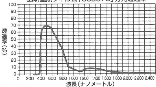
透明遮熱フィルム「SS9070」分光透過率
