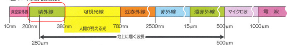
〈図1〉太陽光線波長
